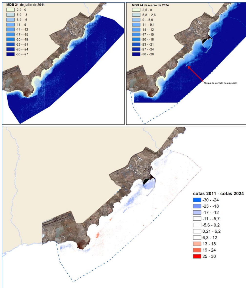
Figura 30: Diferencias (2011-2024) arrojadas por la aplicación IpriSat a partir de imágenes de satélites WorldView. En la parte superior, el modelo batimétrico de cada imagen
