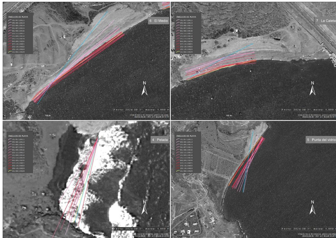
Figura 47: Cambios en la orientación en el eje de las playas en 2024
