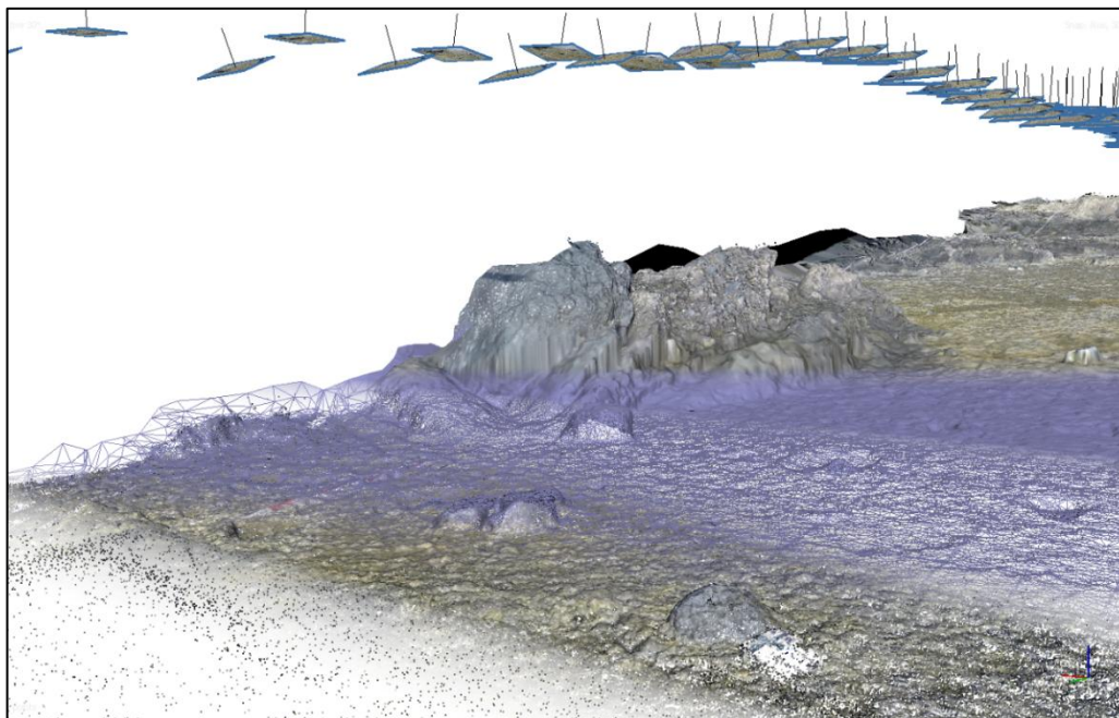
Figura 89: Fases de construcción del modelo 3D a partir de fotogramas extraídos del vídeo. Desde la esquina inferior izquierda hasta la superior derecha, nube de puntos, nube densa de puntos, malla de triangulación, modelo coloreado, modelo texturizado
