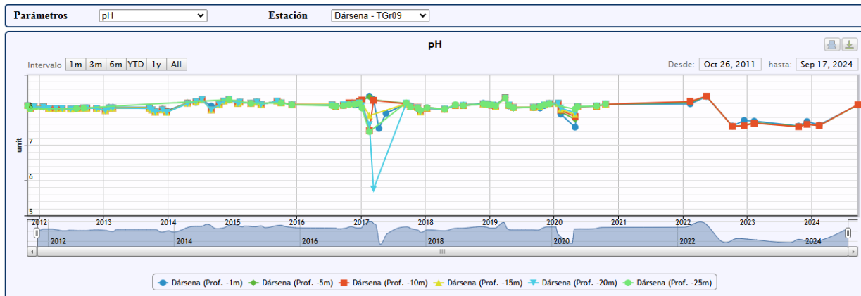
Figura 52: Registro del pH en la estación Dársena (TGr09) (2012-2024)
