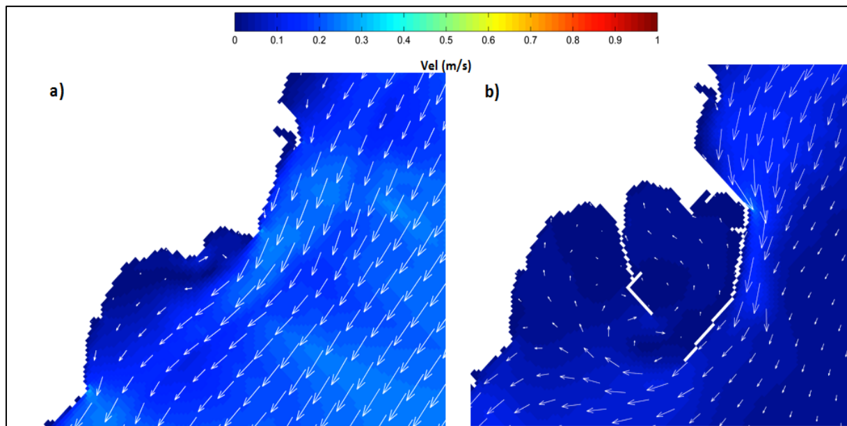
Figura 21: Ejemplo del campo de corrientes promediadas en profundidad en las cercanías del Puerto de Granadilla, en un instante del periodo de simulación (marea vaciante): a) previo; b) posterior
