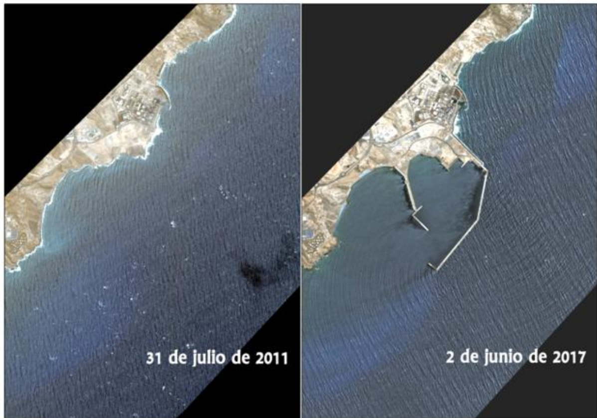
Figura 22: Efecto de las obras de abrigo en el régimen de olas y en su incidencia en la costa. Se aprecian cambios en la dirección y en la energía de las olas, visibles en escenas satelitales
