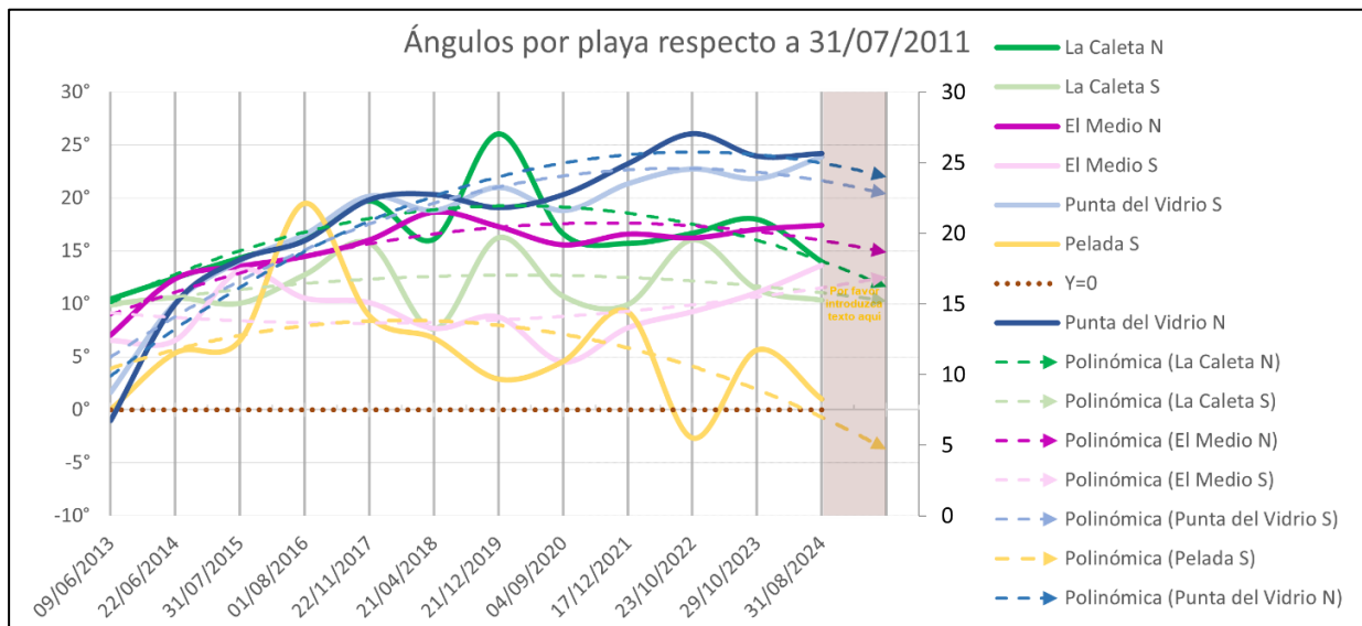
Figura 48: Evolución de los ángulos de basculamiento. Se ha sombreado la proyección a un año vista de la tendencia, calculada con un polinomio cuadrático.
