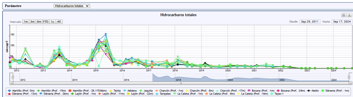
Figura 64: Evolución de hidrocarburos totales 2011-2024 en la costa de Granadilla
