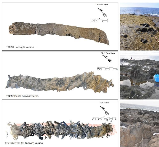
Figura 90: Reconstrucciones de los transectos de TGr16, TGr17 y TGr12b. A la derecha, una instantánea de las orografías.
