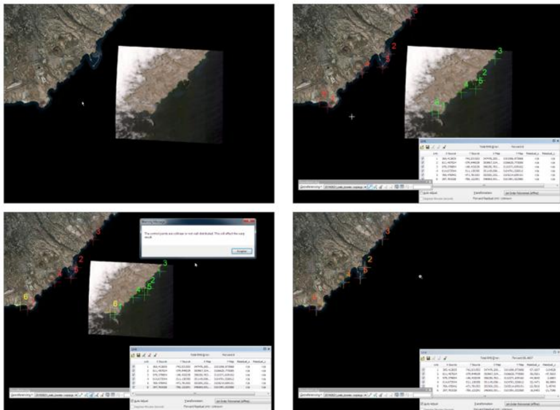
Figura 24: Ejemplo de georreferenciación. Puntos de control y resultado final de la técnica sobre el mapa de la IDE Canarias Ortoexpress del Gobierno de Canarias
