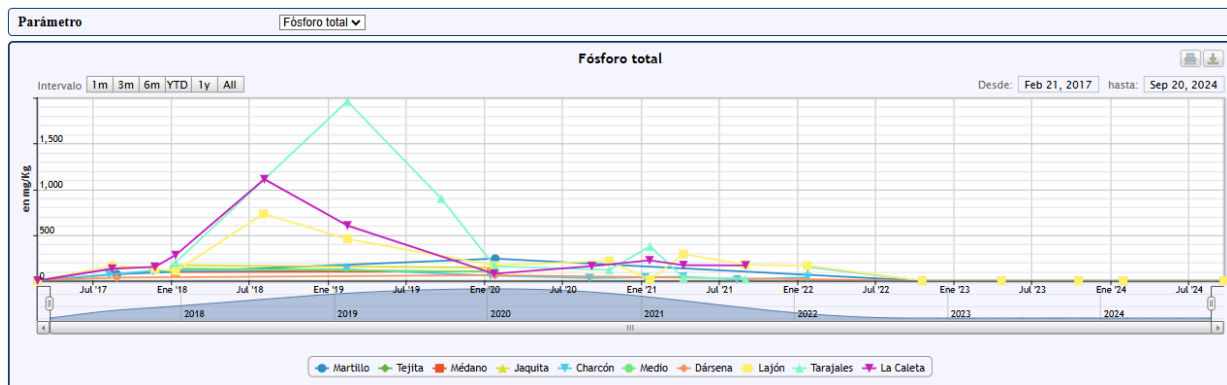
Figura 80: Variación temporal (2011-2024) del fósforo total en las estaciones en Granadilla
