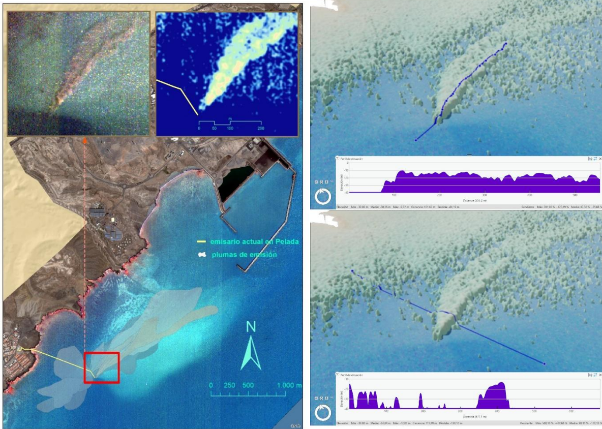
Figura 31: Pluma de emisión de aguas fecales en Pelada a través de un emisario submarino.
