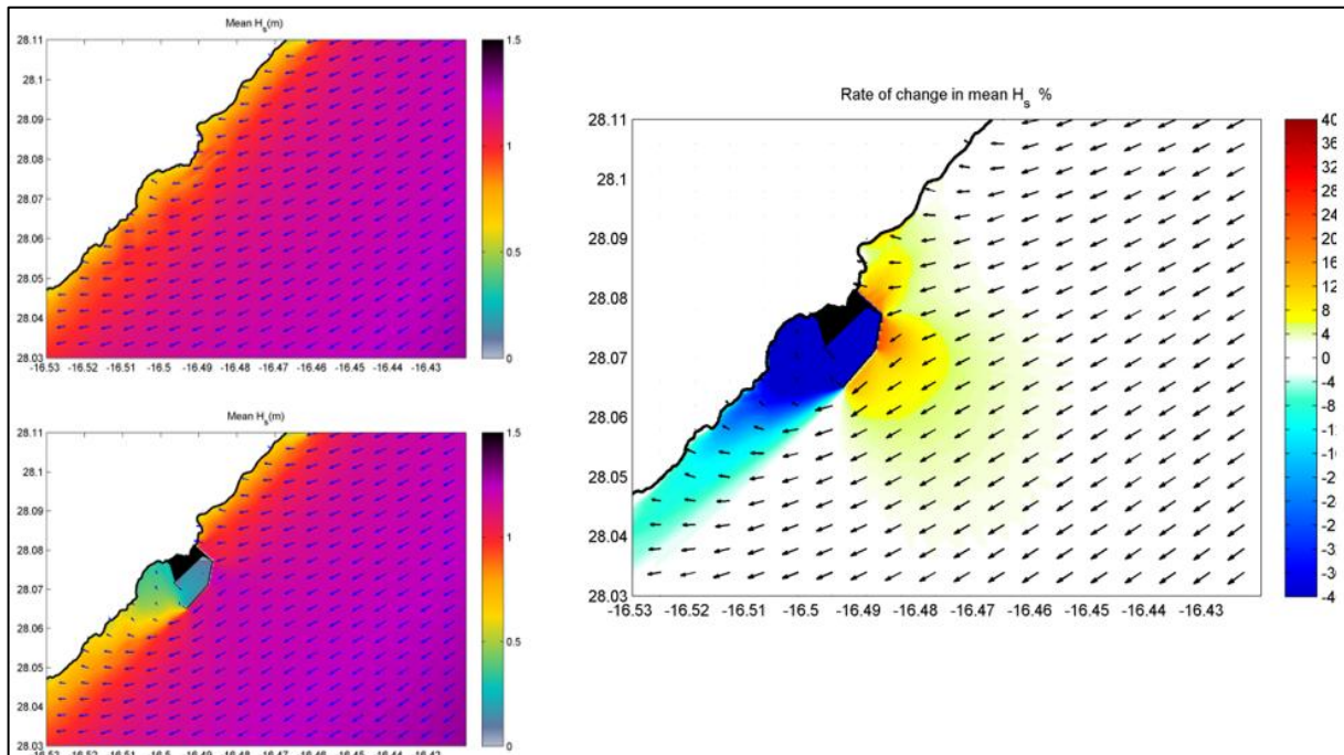
Figura 20: Cambios en el oleaje inducidos. A la izquierda: dirección, sentido (pequeños vectores) y altura significativa media ( H_s ) de las olas antes y después. A la derecha: variación de H_s tras la construcción del puerto. IHC, 2012
